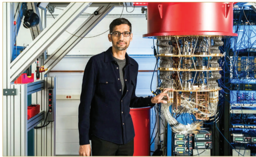
الحاسوب الكمي
